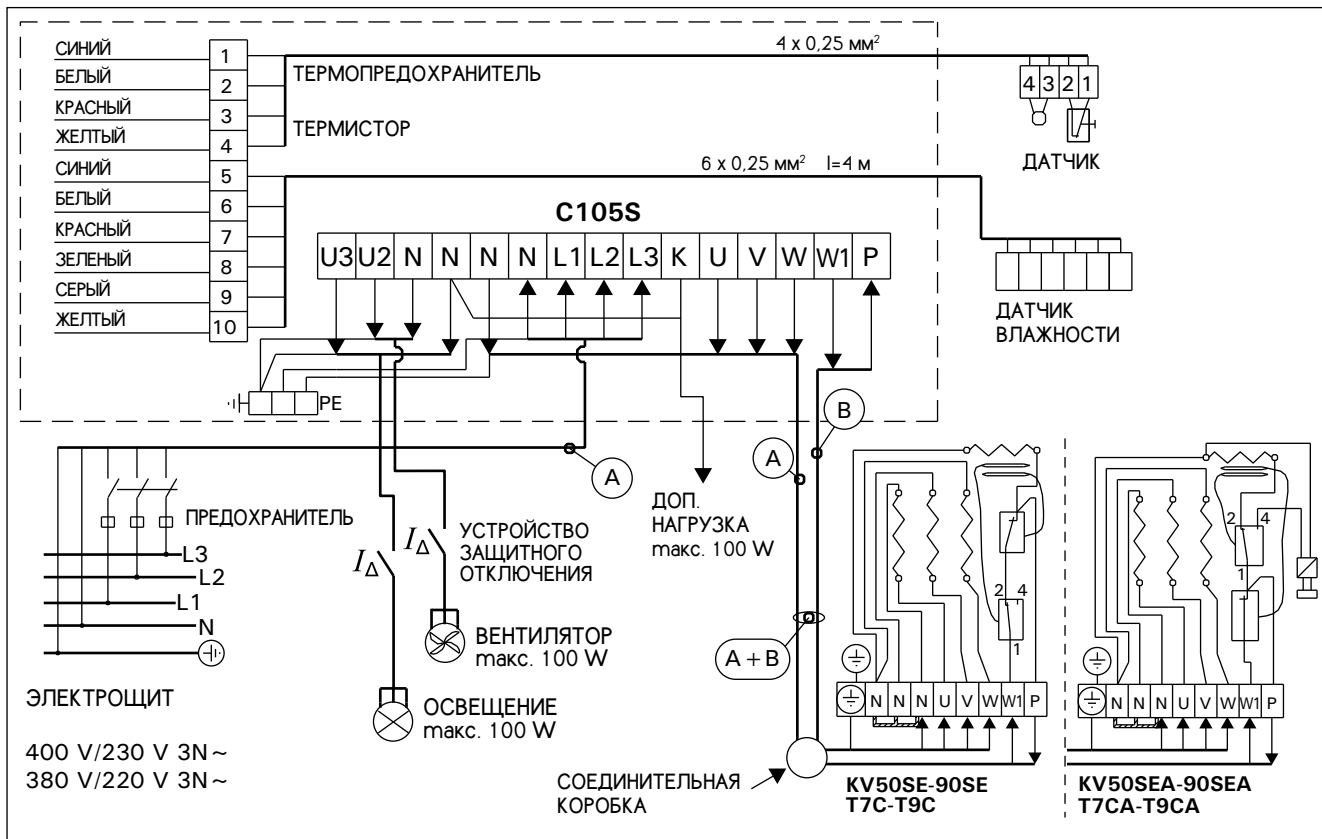
Рисунок 11. 3-фазная сеть
